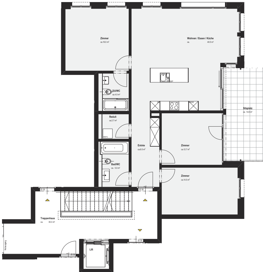
Grundriss Wohnung
